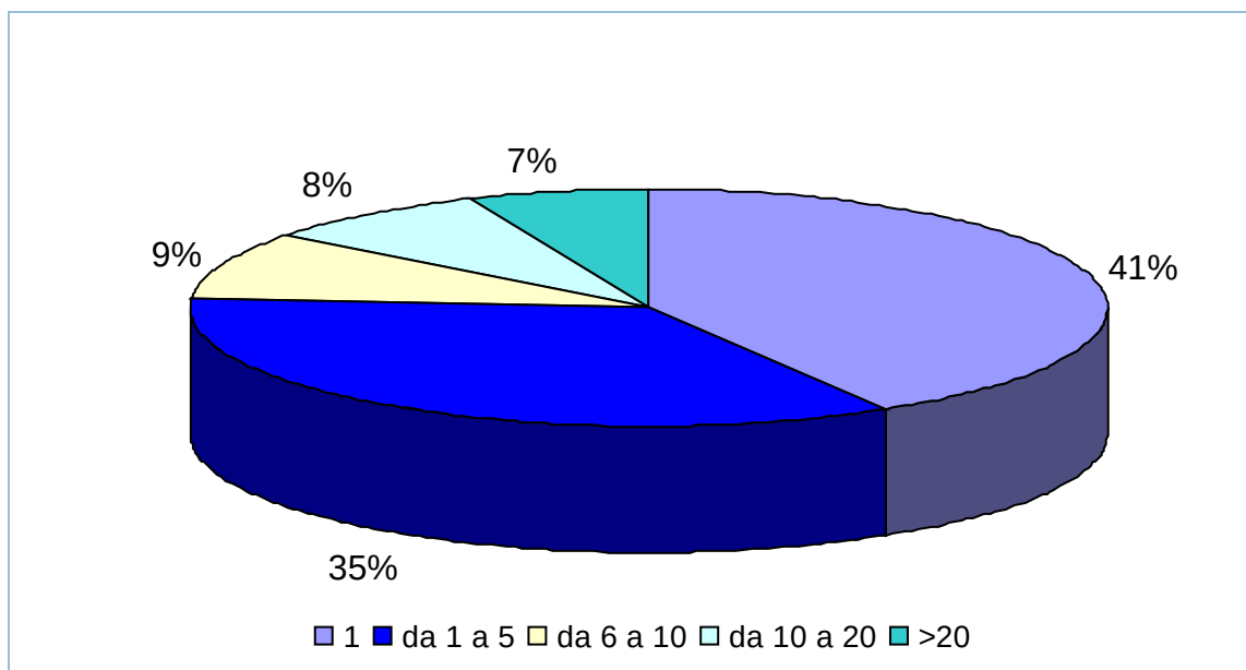
Figura 14.17: Numero di sinkholes per area suscettibile
