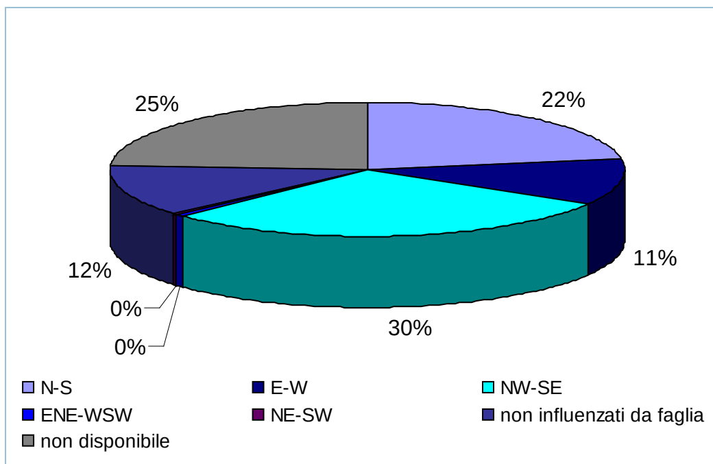
Figura 14.15: Direzioni di faglia
