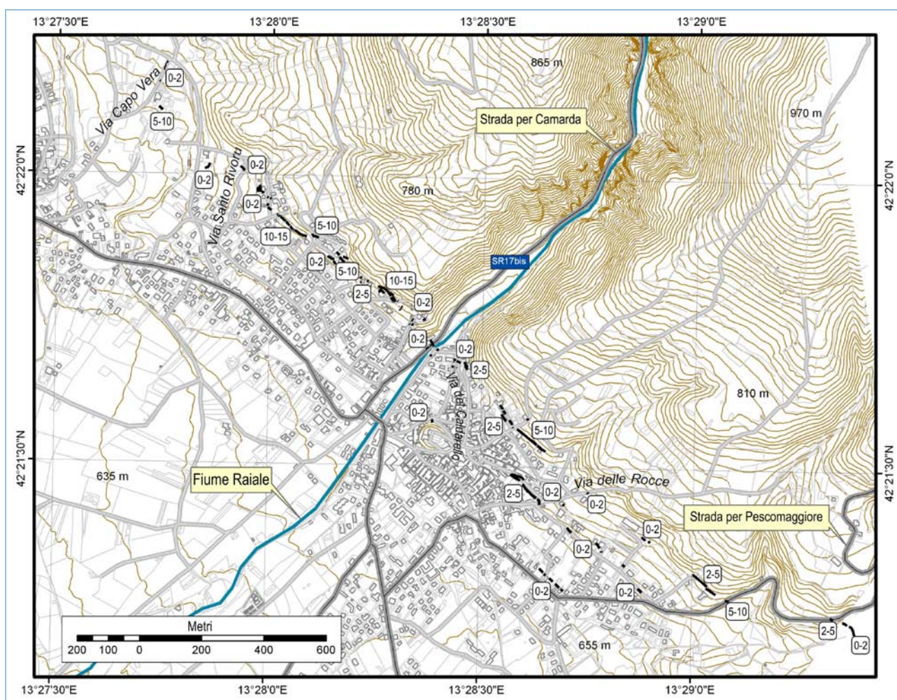
Figura 14.2: Distribuzione areale delle rotture prodotte dall'evento di fagliazione superficiale del 6 Aprile 2009 nella zona di Paganica
