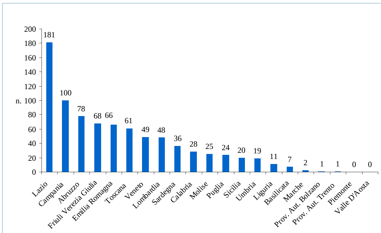
Figura 14.11: Distribuzione dei sinkholes nelle regioni italiane
