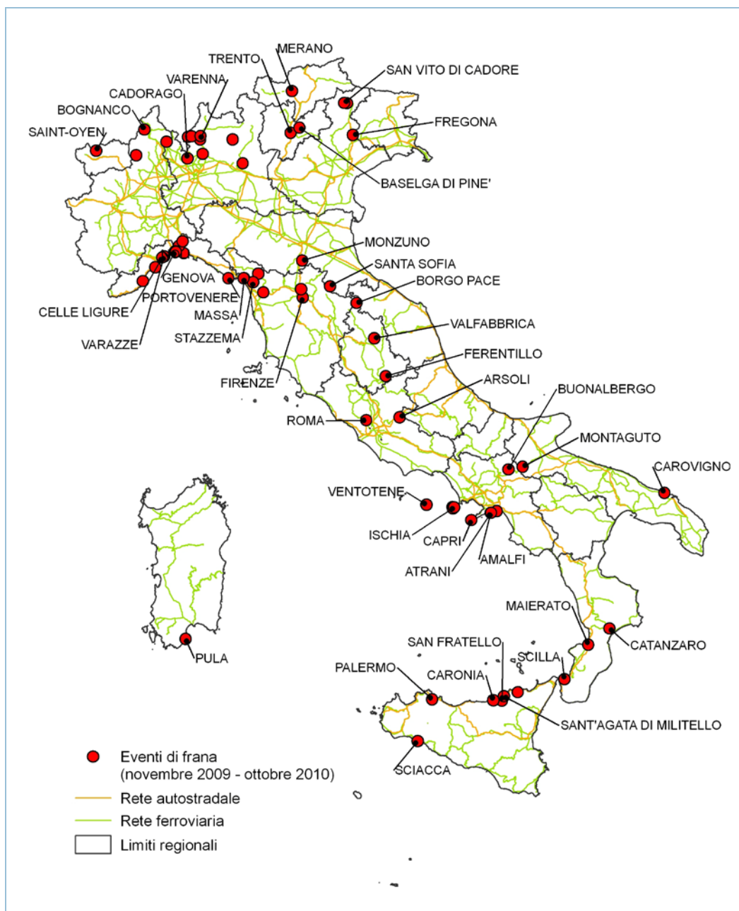
Figura 14.10: Principali eventi di frana nel periodo novembre 2009 – ottobre 2010
