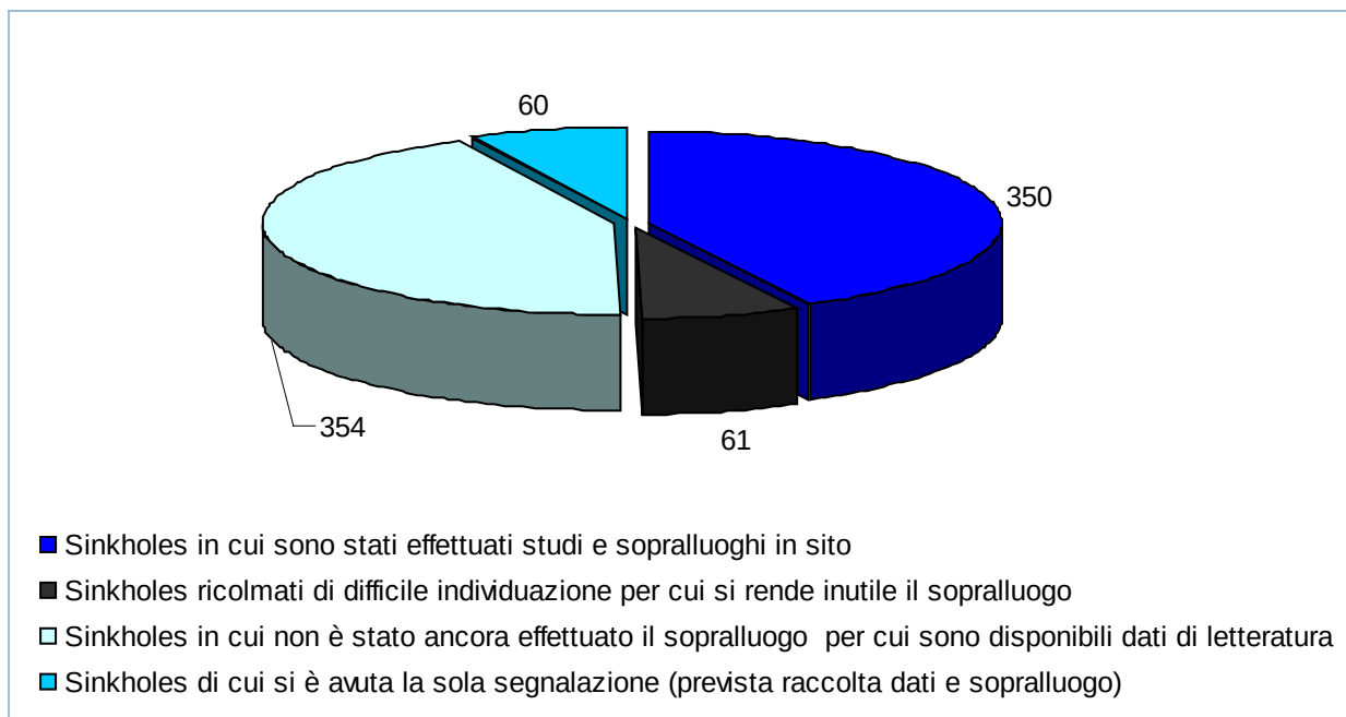
Figura 14.12: Tipologia di dati raccolti
