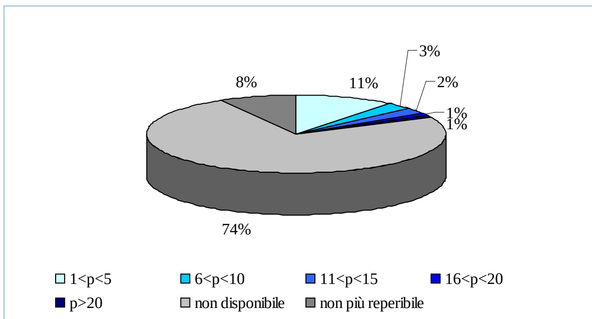
Figura 14.18: Classi di profondità dei sinkholes (m)
