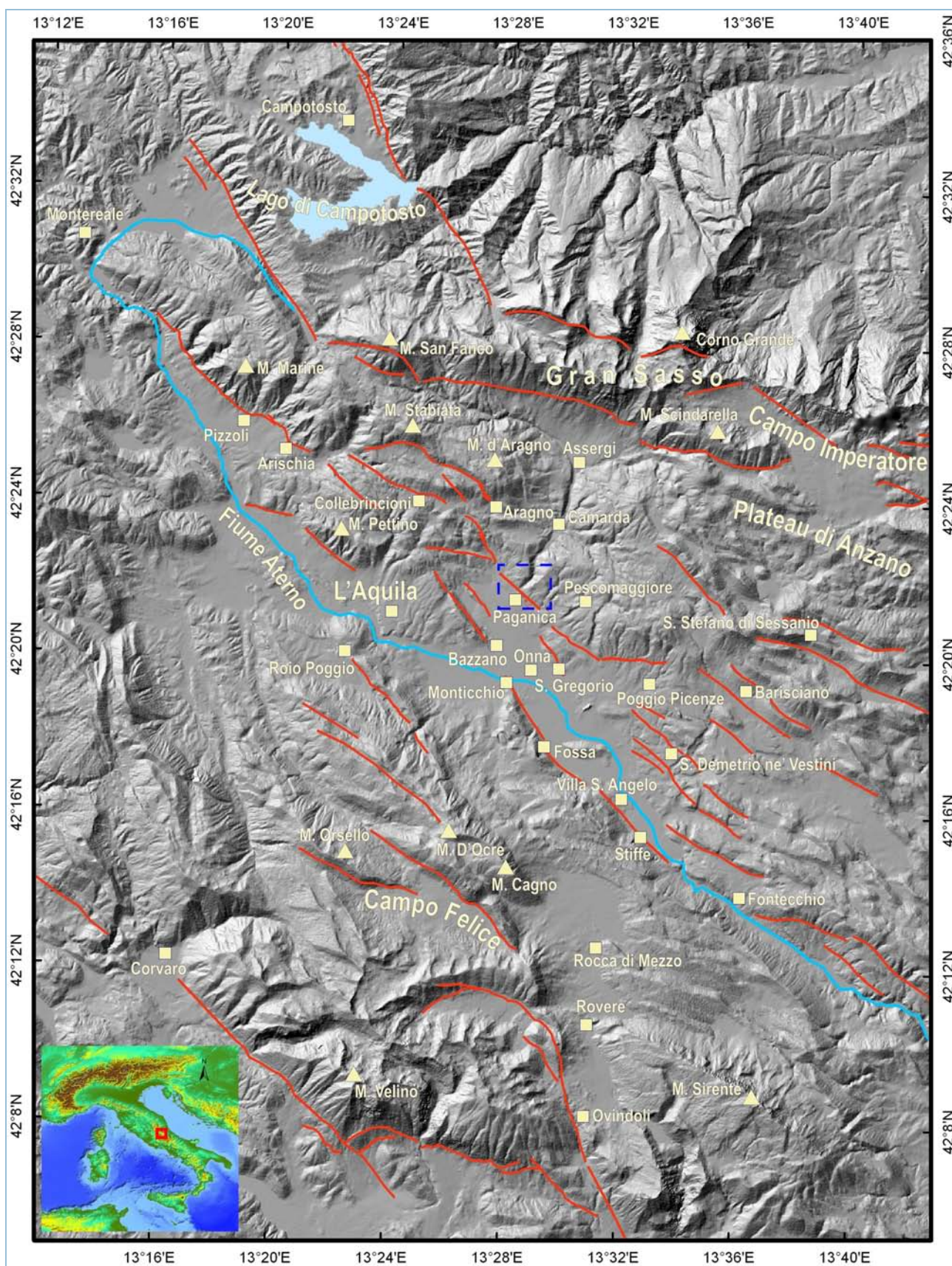
Figura 14.1: Carta delle faglie capaci nell'area abruzzese
