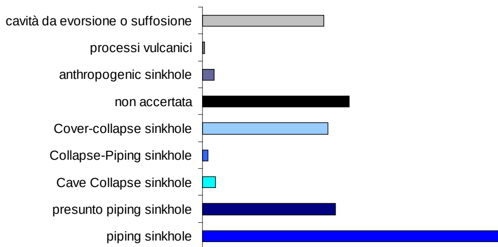
Figura 14.20: Tipologia di sprofondamento
