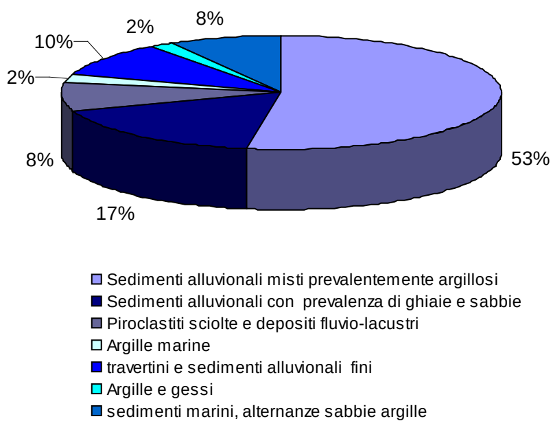
Figura 14.14: Tipologia dei sedimenti di copertura
