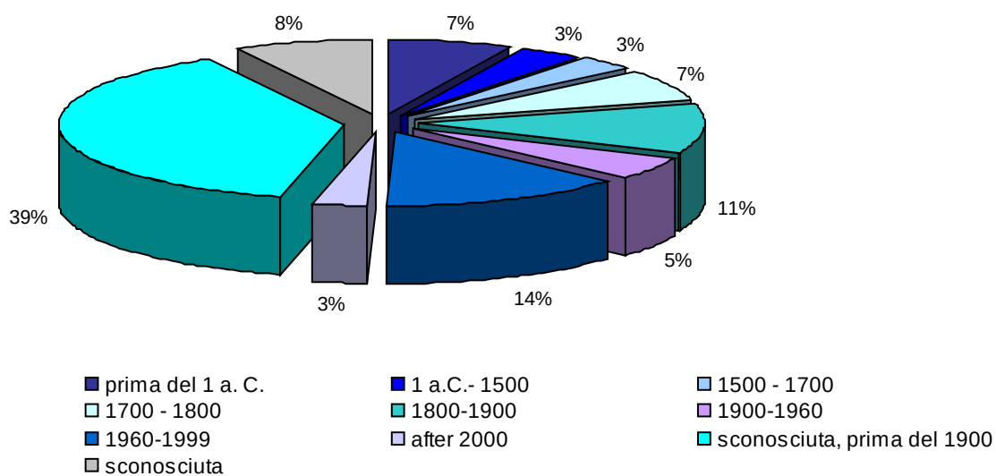
Figura 14.19: Periodo di formazione
