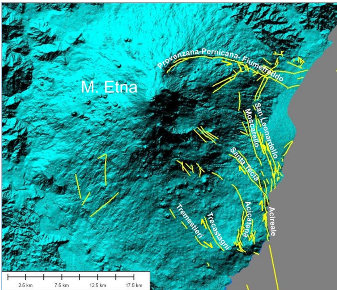
Figura 14.4: Modello digitale del terreno dell'area etnea con riportata la traccia delle faglie capaci. Tra di esse è indicata la faglia di S. Leonardello, alla cui base si è verificata la fratturazione in superficie durante il terremoto del 13/05/09
