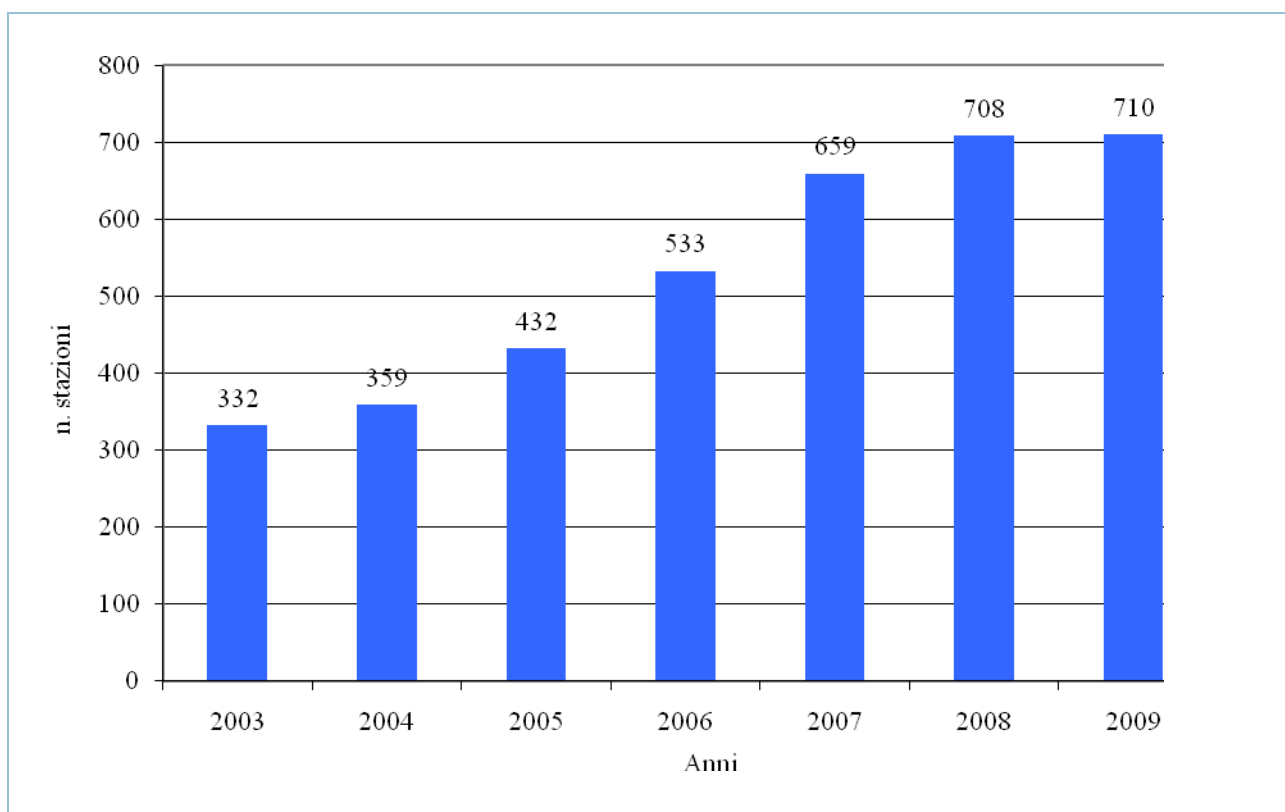
Figura 6.19: Stazioni di rilevamento per la qualità dell'aria
