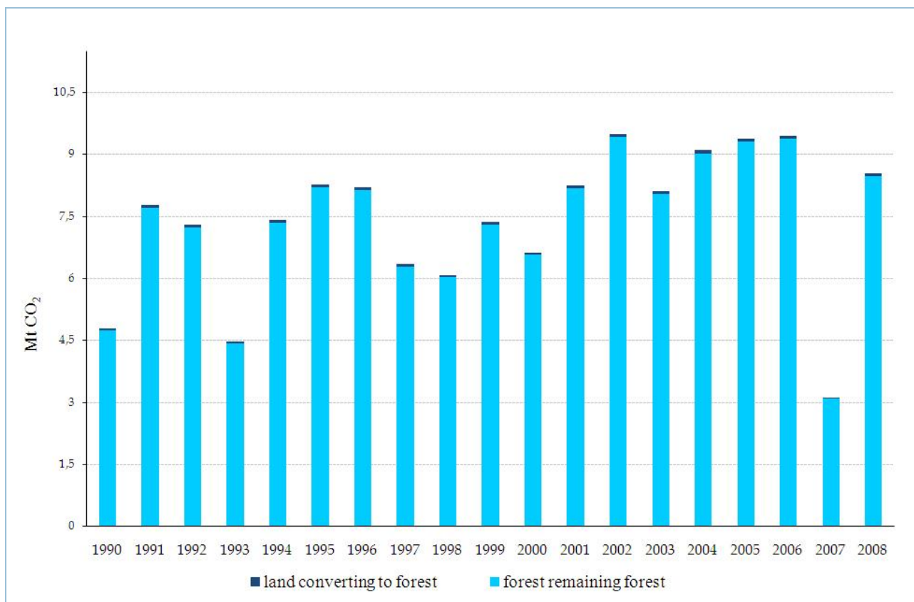
Figura 6.5: Variazioni negli stock di carbonio relativamente alla sola biomassa (epigea e ipogea)
