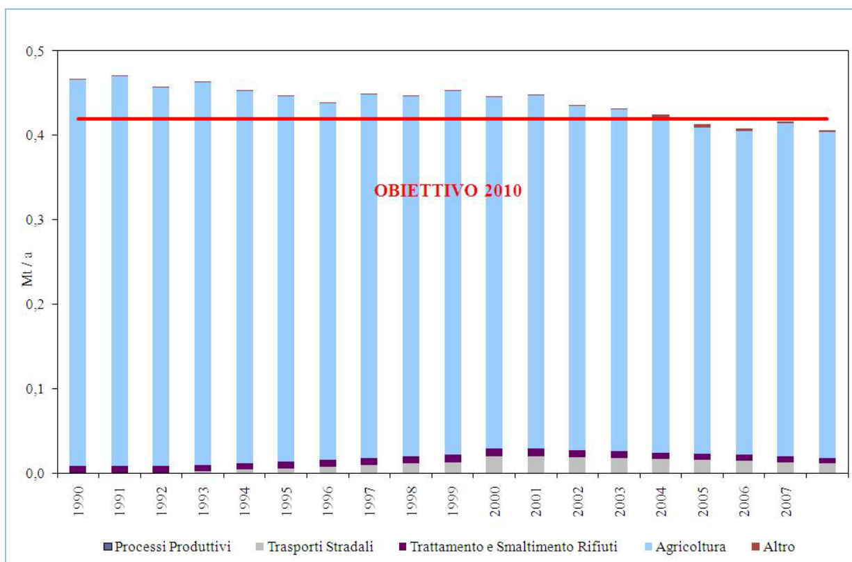
Figura 6.9: Emissioni nazionali di ammoniaca (NH 3 )
