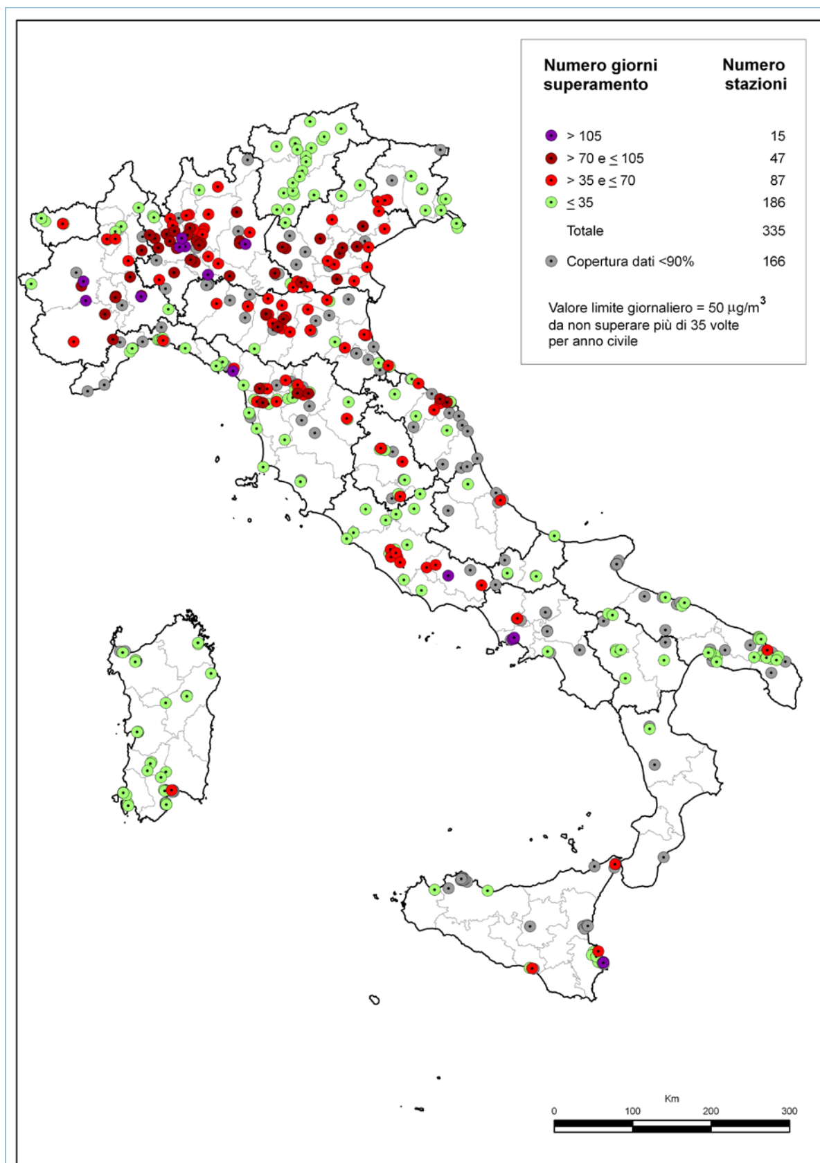
Figura 6.23: PM 10 - Stazioni di monitoraggio per classi del numero giorni di superamento del valore limite giornaliero ( 50 \mu\text{g}/\text{m}^3 da non superare più di 35 volte per anno civile) (2009)
