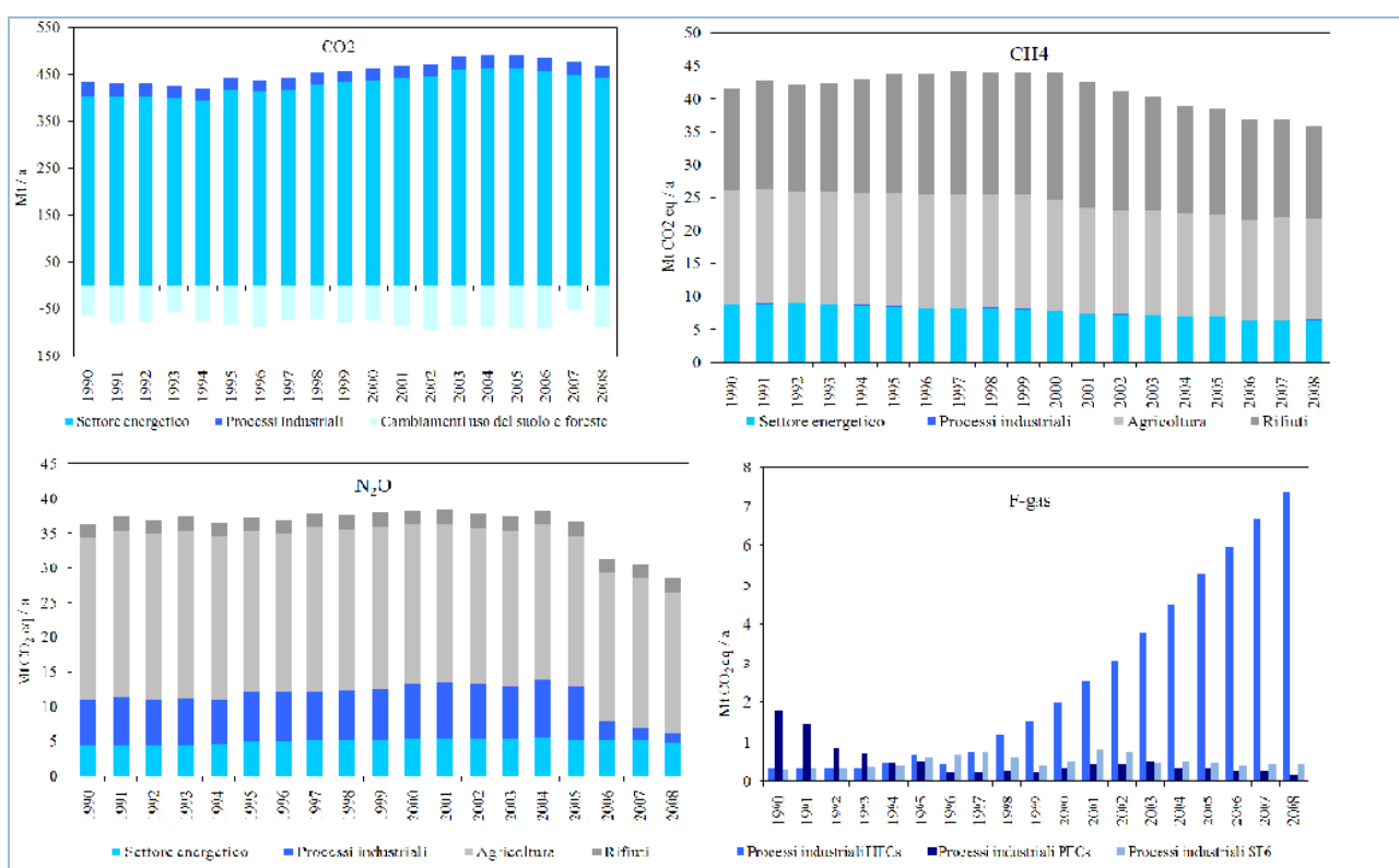
Figura 6.1: Emissioni nazionali complessive di gas serra
