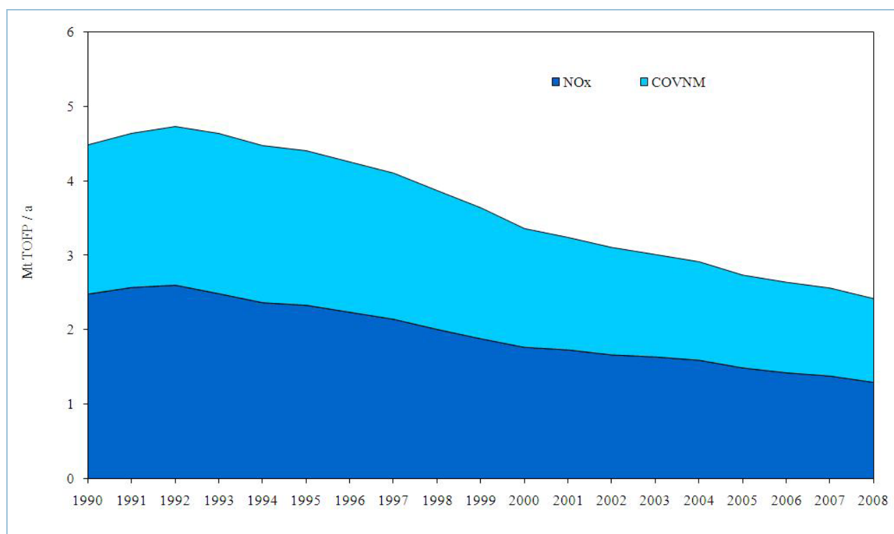
Figura 6.13: Emissioni nazionali complessive di ossidi di azoto (NO x ) e composti organici volatili non metanici (COVNM)
