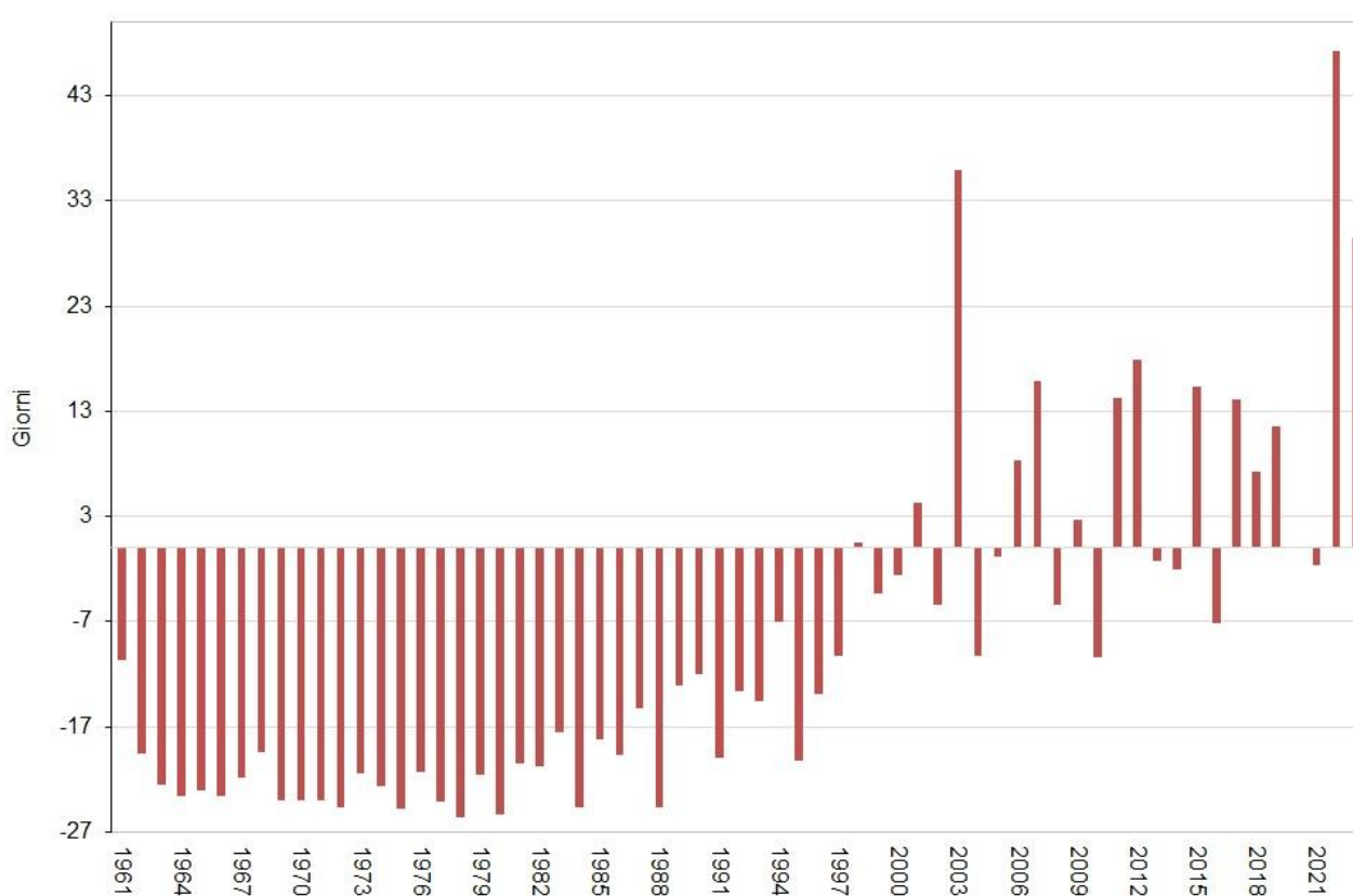
Serie delle anomalie medie annuali del numero di giorni con onde di calore (WSDI) in Italia rispetto al valore normale 1991-2020
