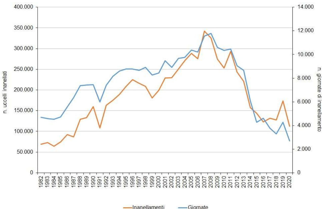
Andamento annuale del numero di uccelli inanellati e delle sessioni di inanellamento espresse in giorni
