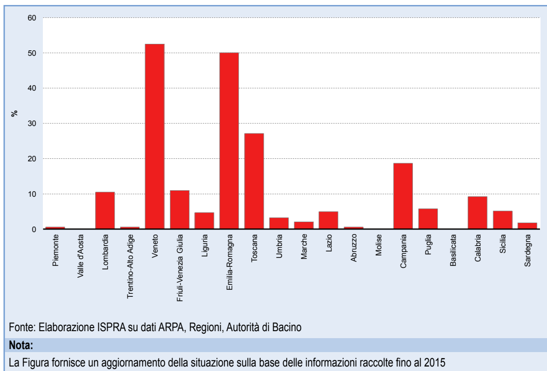
Figura 15.31 : Comuni interessati da subsidenza
