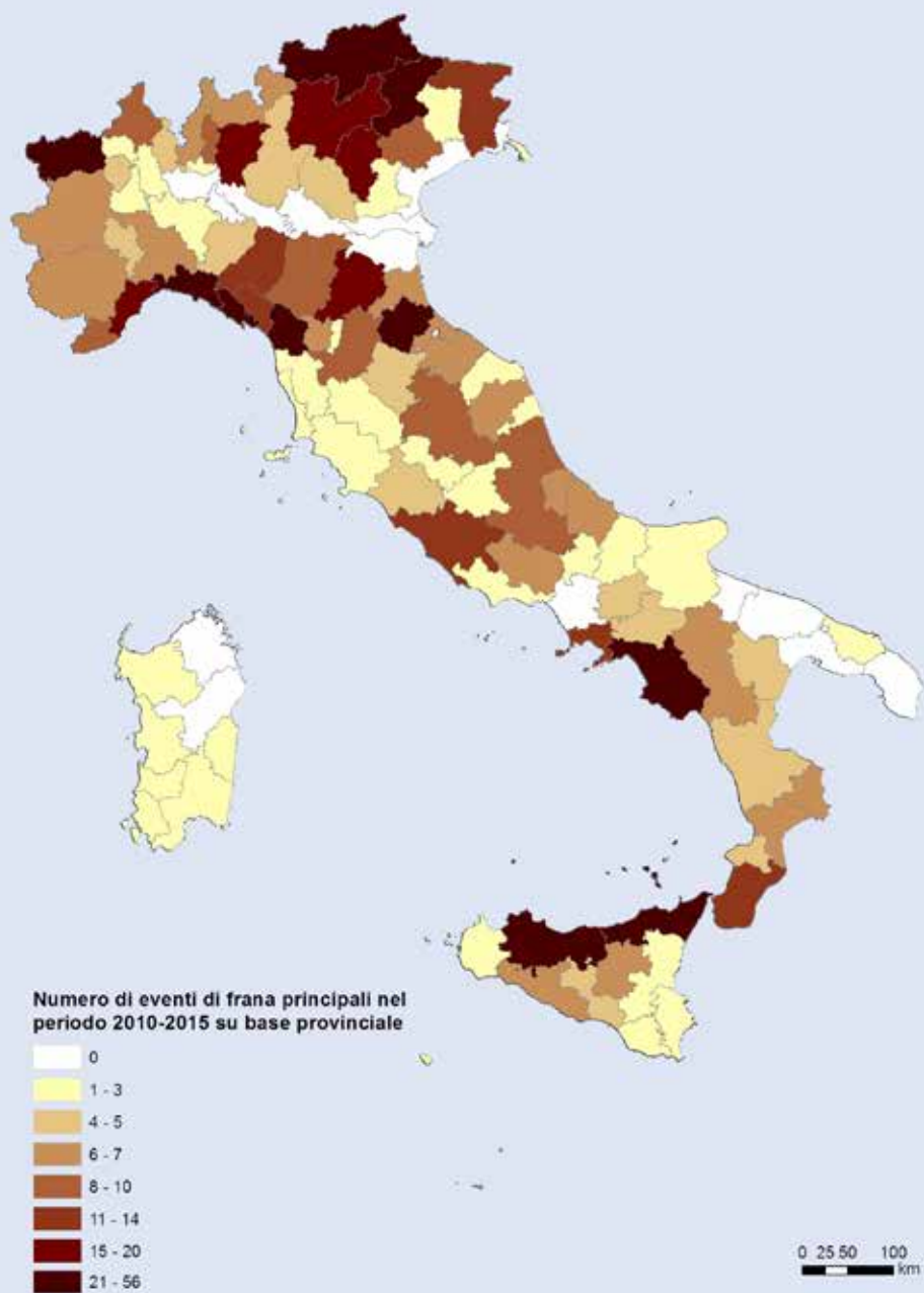
Figura 15.19: Numero di eventi di frana principali nel periodo 2010-2015 su base provinciale
