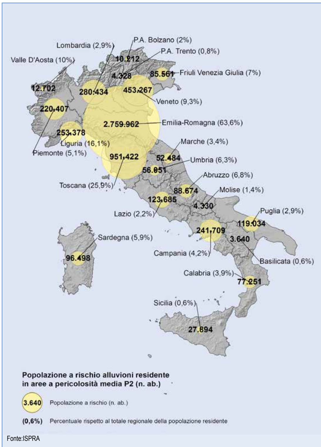
Figura 15.16: Popolazione esposta ad alluvioni con pericolosità media P2 (tempo di ritorno fra 100 e 200 anni) su base regionale (2015)
