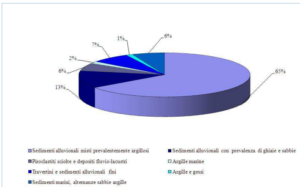
Figura 14.11: Tipologia dei sedimenti costituenti la copertura delle aree suscettibili ai fenomeni di sinkhole naturali
