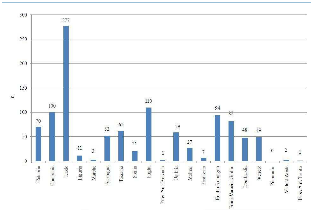
Figura 14.10: Distribuzione dei sinkholes naturali nelle regioni italiane
