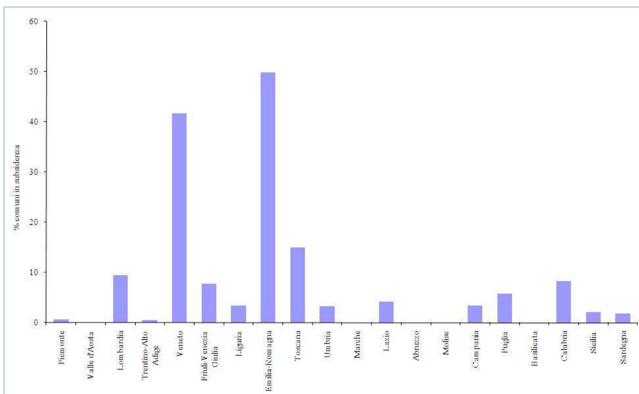
Figura 14.16: Percentuale comuni in subsidenza (2011)
