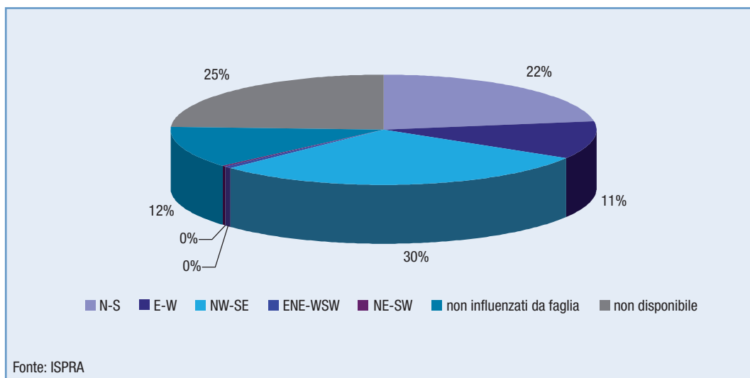
Figura 14.23: Direzioni di faglia relative agli elementi tettonici che influenzano direttamente le cavità
