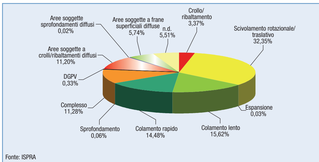
Figura 14.11: Tipologia di movimento dei fenomeni franosi
