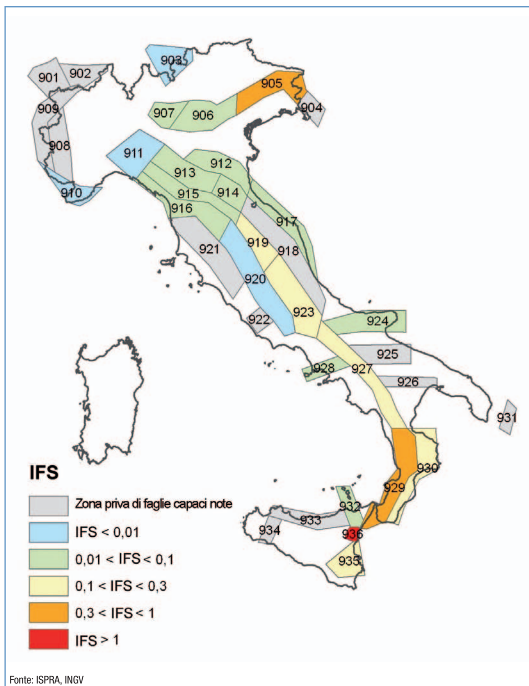
Figura 14.4: Classificazione delle zone sismogenetiche ZS9 in funzione dell'indice IFS
