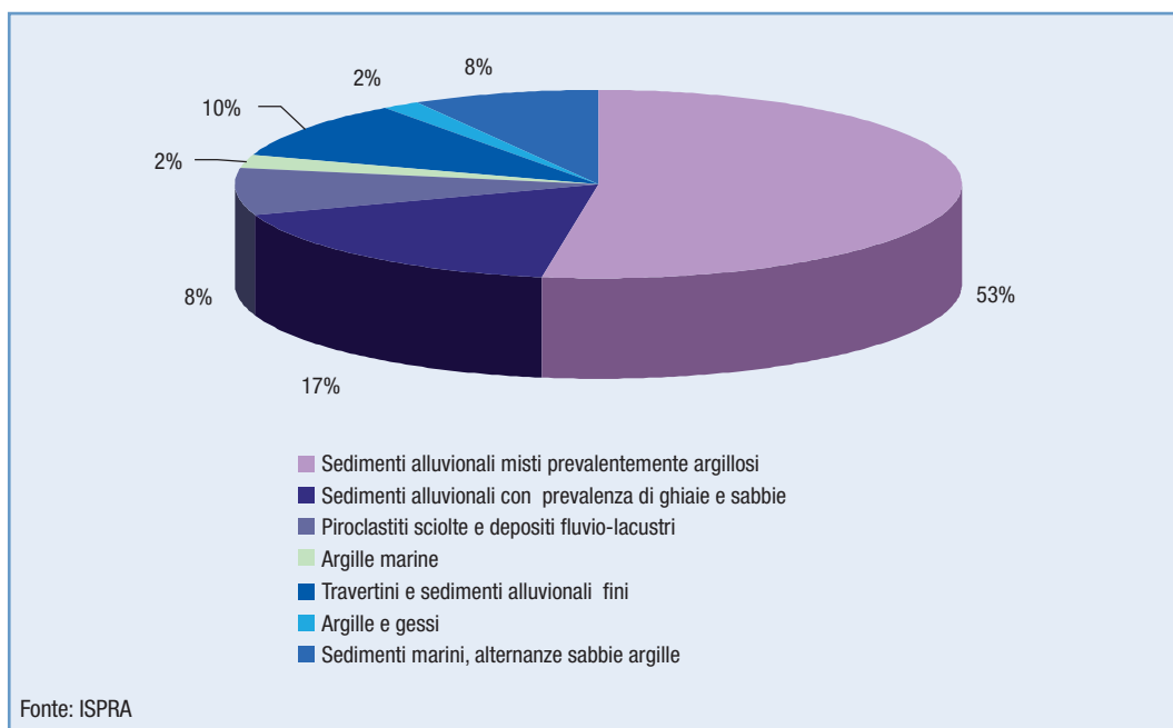
Figura 14.20: Tipologia dei sedimenti di copertura
