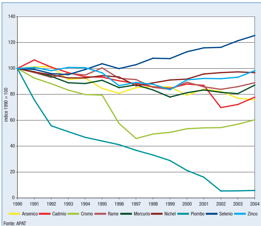
Figura 6.25: Emissioni nazionali di metalli pesanti
