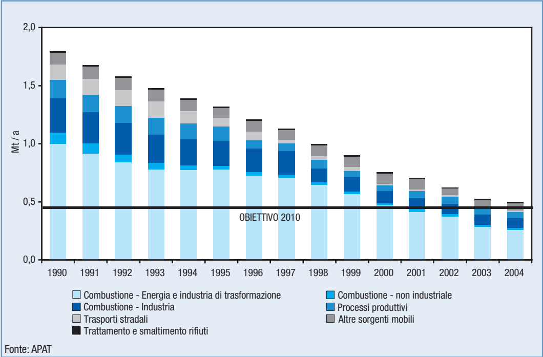
Figura 6.6: Emissioni nazionali di ossidi di zolfo (SO x )
