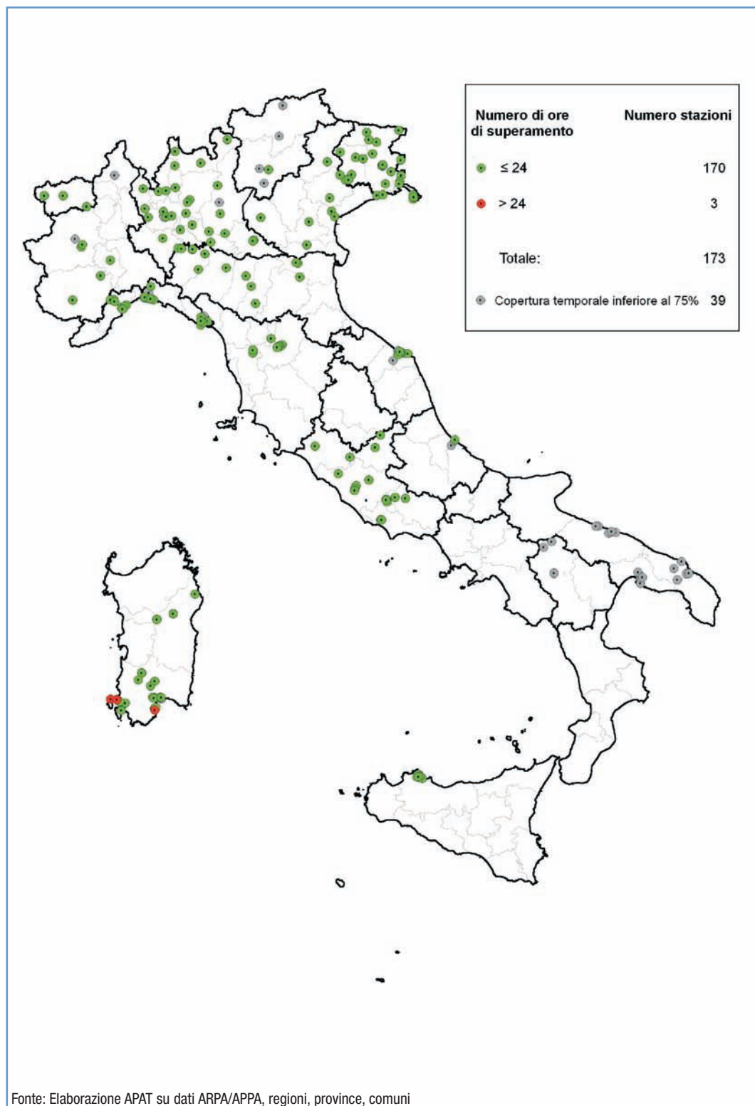
Figura 6.35: SO 2 , stazioni di monitoraggio per classi di ore di superamento del valore orario di 350 µg/m 3 (2004)
