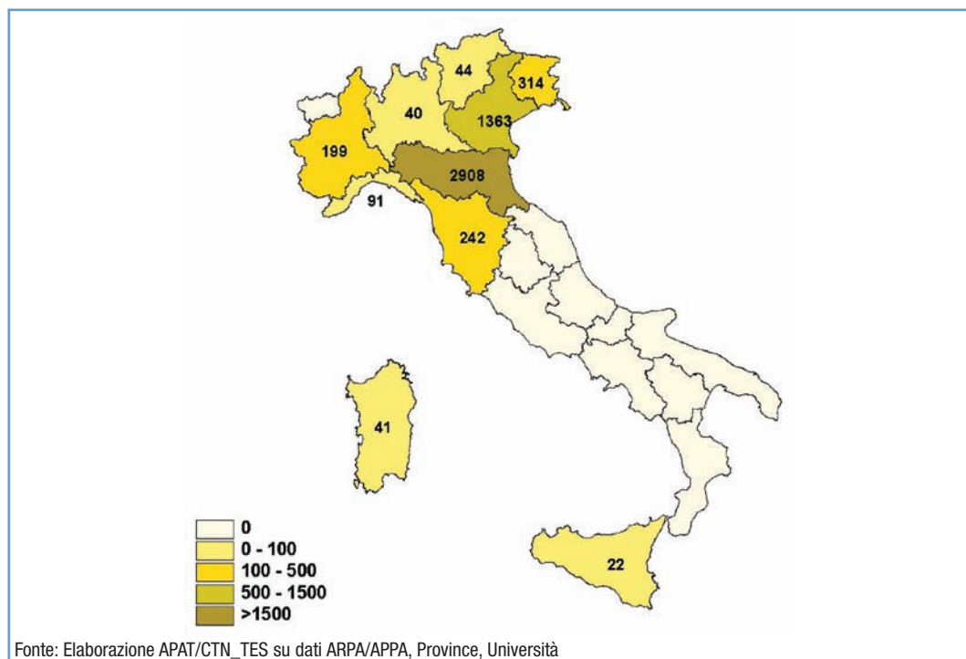
Figura 13.4a: Numero totale di campioni analizzati e densità geografica dei dati (2000)
