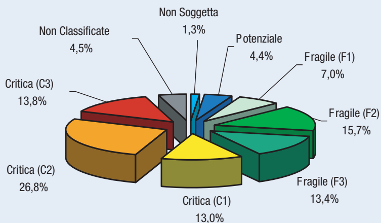
Figura 13.21: Ripartizione delle aree sensibili alla desertificazione in Sardegna (2004)
