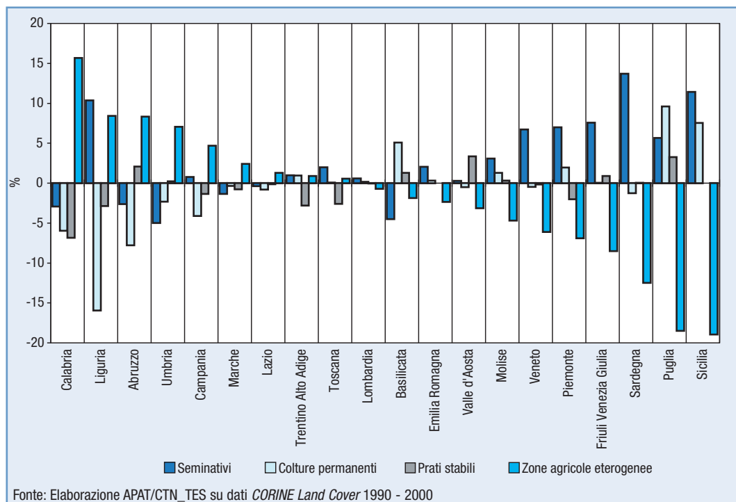
Figura 13.44: Variazione percentuale dell'area agricola per regione (1990-2000)
