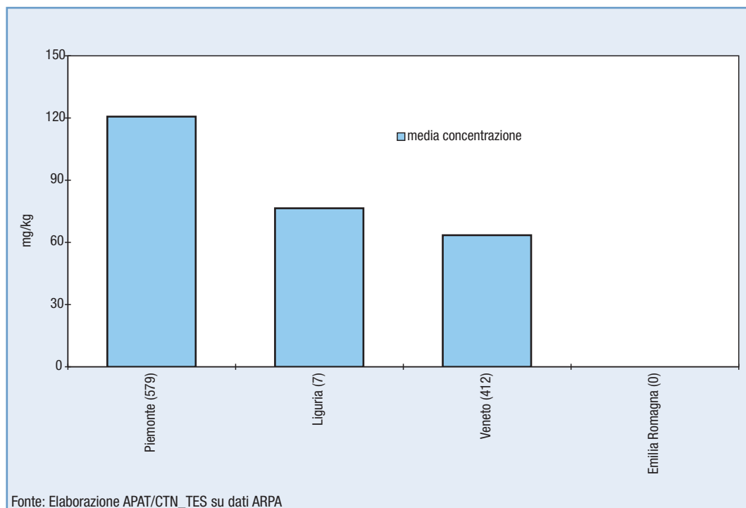
Figura 13.6b: Valori medi relativi alla concentrazione di cromo nei terreni agricoli italiani (rilievi dal 2001)
