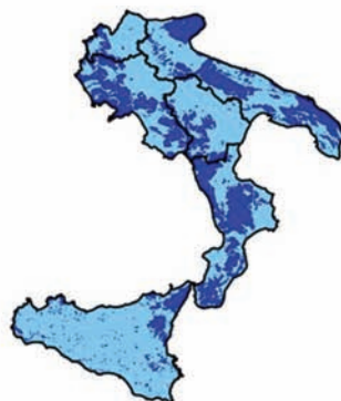
Figura 13.3: Contenuto in percentuale di CO negli orizzonti superficiali dei suoli del Sud Italia (1988-2003)
