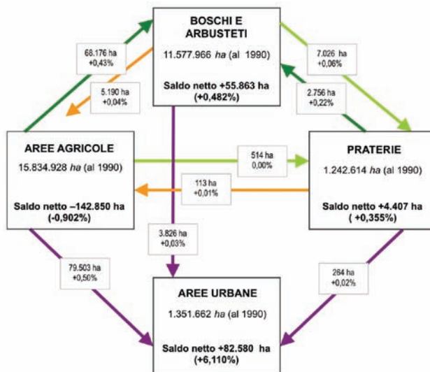
Figura 13.47: Schema delle principali transizioni delle coperture delle terre (1990-2000)
