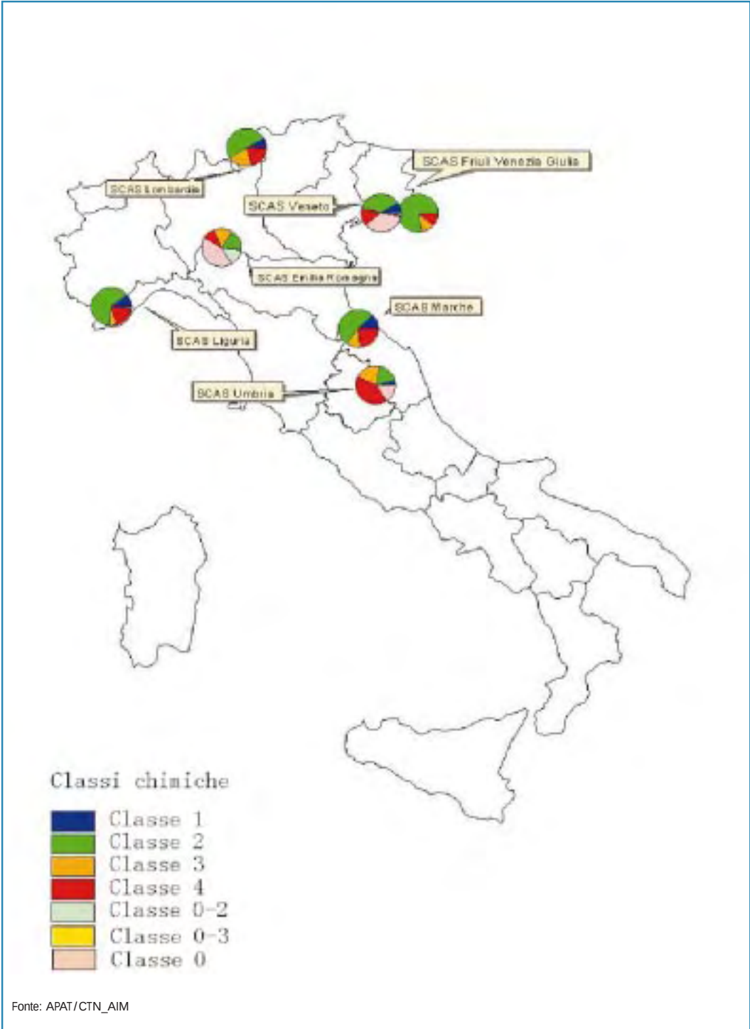
Figura 3.16: Stato qualitativo dei corpi idrici sotterranei, % sul totale dei punti monitorati
