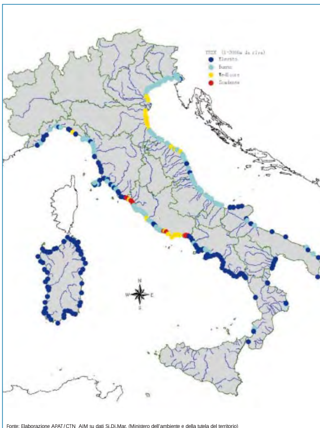
Figura 3.2: TRIX, classi di qualità sulle medie biennali 1997-1998 nelle acque costiere comprese tra 500 e 3000 m da riva
