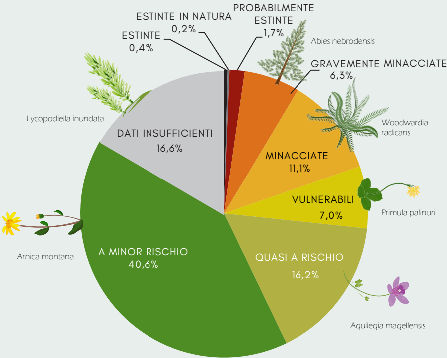
Figura 31: Livello di minaccia della flora vascolare italiana: ripartizione percentuale nelle categorie IUCN di rischio di estinzione delle 2.430 piante vascolari valutate (2020)
