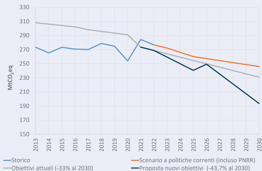
Figura 5: Trend e proiezioni delle emissioni di gas serra soggette al regolamento "Effort Sharing"
