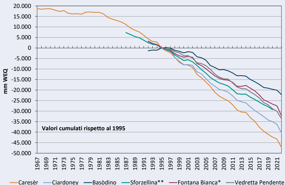
Figura 3: Bilancio di massa cumulato di alcuni ghiacciai italiani
